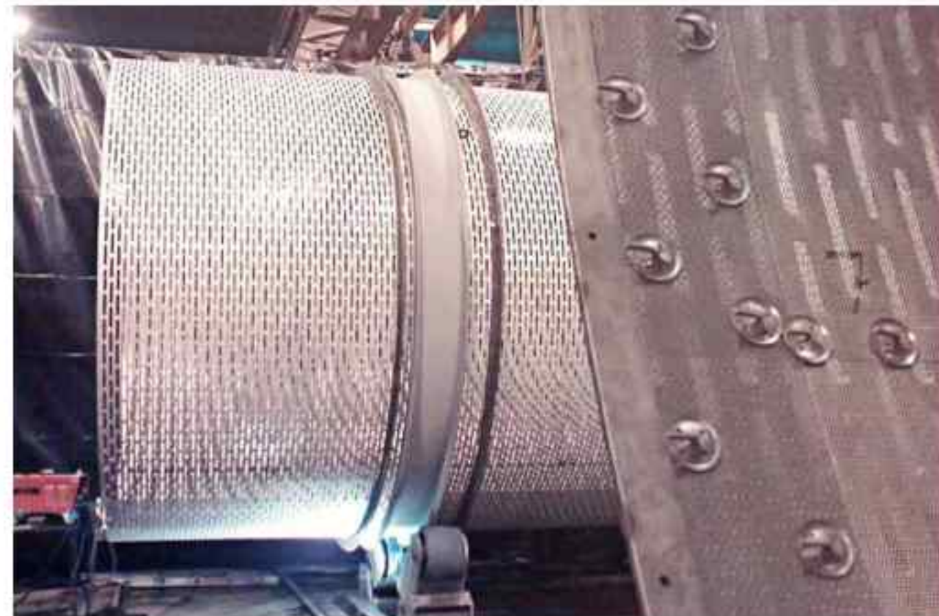
FABRICACIÓN EN INOXIDABLE DE LOS ABSORBEDORES R201 & R202 - AIR LIQUIDE
