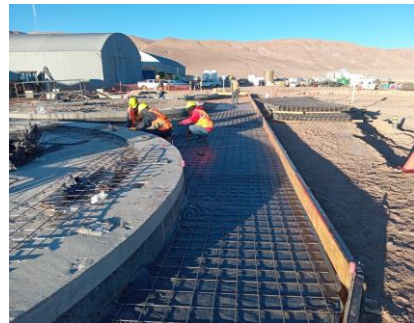
RINCÓN Ltd. 3 kTPA Rapid Plant – Fundaciones Edificios y Equipos | 2023 BSD-GECO
